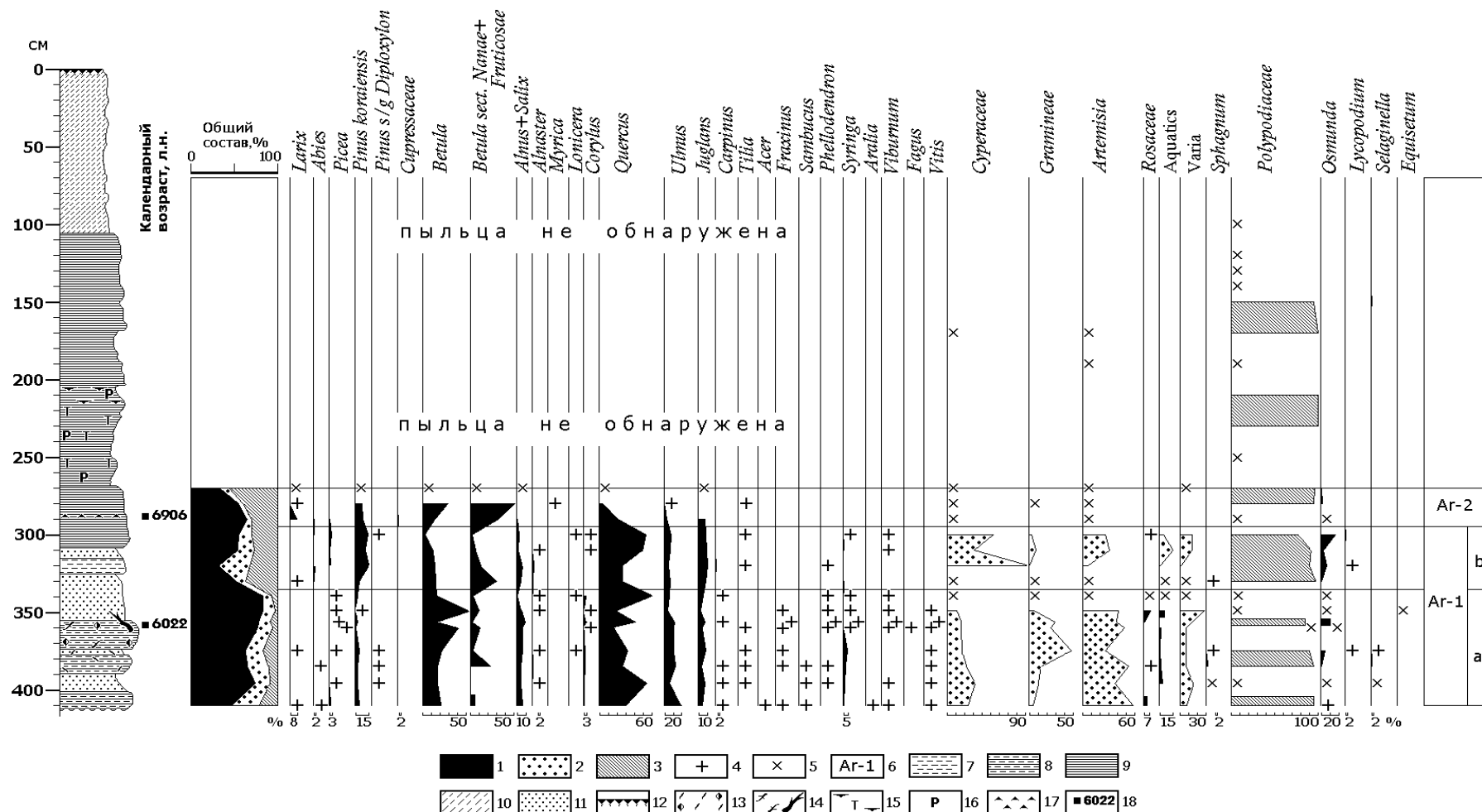
Рис. 3. Спорово-пыльцевая диаграмма отложений разреза «Арзамавка»
