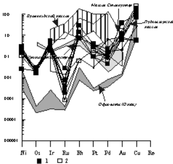
Рис. 27. Распределение ЭПГ в породах Лукинского массива, нормализованные по хондриту С, (Donogh, Sun, 1995), в сравнении с эталонными объектами.
