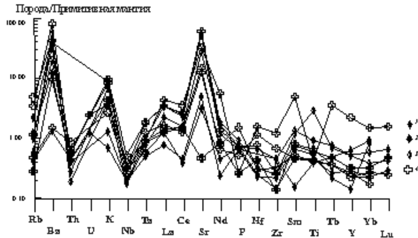
Рис. 6. Нормированные по примитивной мантии (Sun, Donogh, 1989) спектры распределения малых элементов в породах массива Маристый. Условные обозначения: 1 - ультрамафиты, 2 - пироксениты, 3 - габброиды; 4 - анортозиты
