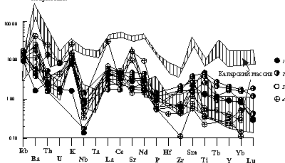
Рис. 5. Нормированные по первичной мантии (Sun, Donogh, 1989) спектры распределения малых элементов в породах Хорогочинского массива. Условные обозначения: 1 - ультрамафиты; 2 - пироксениты; 3 - габброиды; 4 - анортозиты
