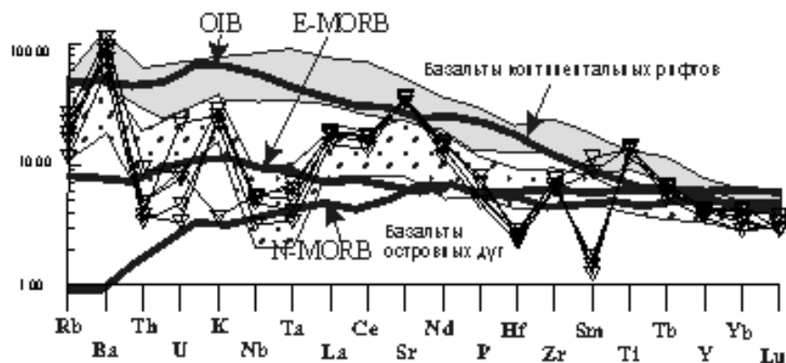
Рис. 17. Нормированные по примитивной мантии (Sun, Donogh, 1989) спектры распределения малых элементов в габброидах массива Ульдегит. Поля типичных составов базальтов островных дуг, базальтов континентальных рифтов по (Великославинский, Глебовицкий, 2005). Состав N-MORB, E-MORB, OIB - по (Sun, Donogh, 1989).
