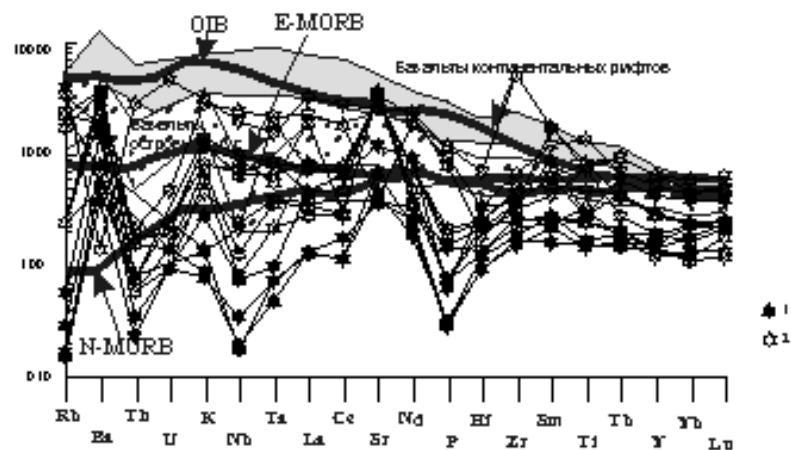
Рис. 18. Нормированные по примитивной мантии (Sun, Donogh, 1989) спектры распределения малых элементов в породах массива Чек-Чикан. Условные обозначения см. рис. 11: 1 - пироксениты, 2 - габброиды;
