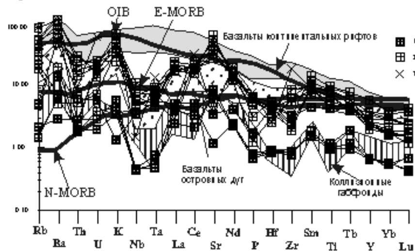
Рис.21. Нормированные по примитивной мантии (Sun, Donogh, 1989) спектры распределения малых элементов в породах массива Петропавловский. Поля типичных составов базальтов островных дуг, базальтов континентальных рифтов по (Великославинский, Глебовицкий, 2005). Состав N-MORB, E-MORB, OIB - по (Sun, Donogh, 1989). Условные обозначения: 1 - пироксениты; 2 - габброиды; 3 - диориты.
