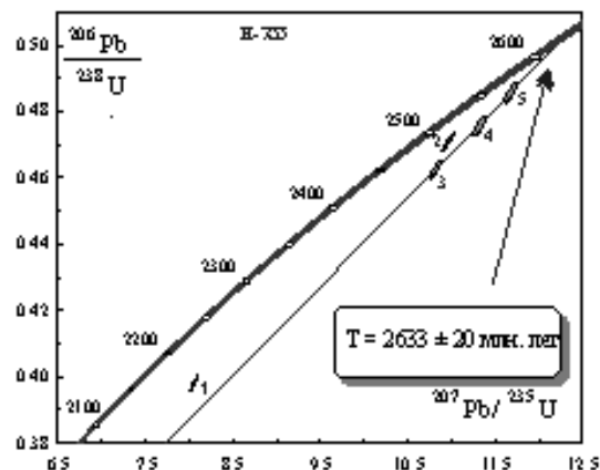
Рис. 2 Диаграмма с конкордией для цирконов из анортозитов Хорогочинского массива
