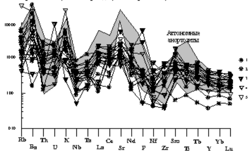
Рис. 9. Нормированные по примитивной мантии (Sun, Donogh, 1989) спектры распределения малых элементов в породах массивов Орогжан и Сергачинский. Поле автономных анортозитов по материалам Н.В Бердникова. Условные обозначения массивов Орогжан - 1-2, Сергачинского - 3-5: 1 - габбро, 2 - габбро-анортозиты; 3 - пироксениты, 4 - габброиды, 5 - анортозиты
