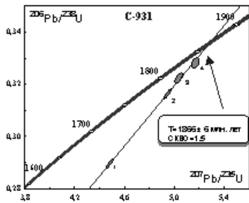
Рис. 8. Диаграмма с конкордией для цирконов из анортозитов Сергачинского массива
