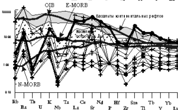
Рис.14 Нормированные по примитивной мантии (Sun, Donough, 1989) спектры распределения малых элементов в породах Ильдеуского массива. Условные обозначения см. рис.11: 1 - перидиты, плагиовериты, 2 - пироксениты, 3-габброиды
