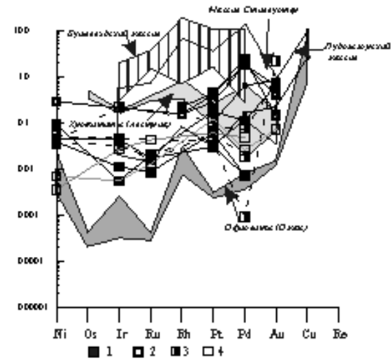
Рис. 28. Распределение ЭПГ в породах Веселинского массива, нормализованные по хондриту С, (Donogh, Sun, 1995), в сравнении с эталонными объектами.
