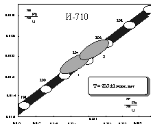
Рис.16. Диаграмма с конкордией для цирконов из габбронорита массива Чек-Чикан
