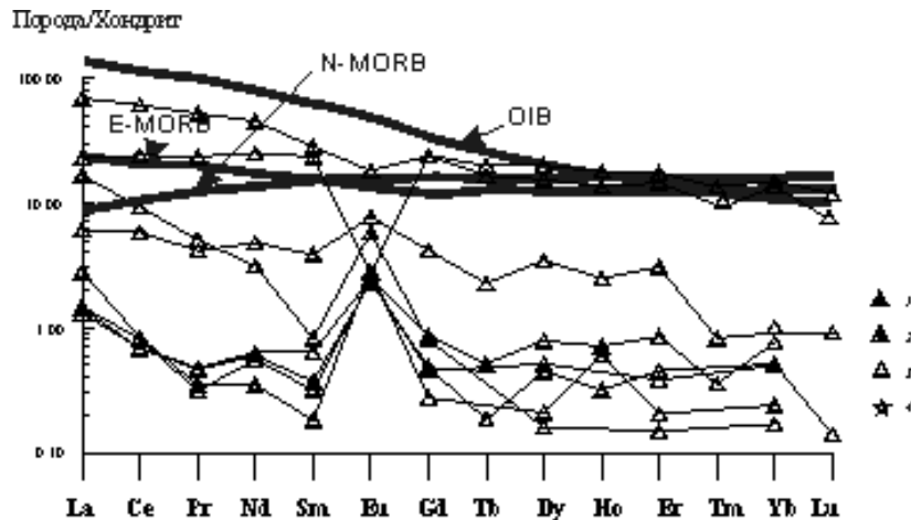
Рис. 7. Нормированные по хондриту C (Donogh, Sun, 1995) спектры распределения РЗЭ в породах массива Баладек. Состав N-MORB, E-MORB, OIB - по (Sun, Donogh, 1989). Условные обозначения породы: 1 - ультрамафиты; 2 - пироксениты; 3 - габброиды; 4 - анортозиты;
