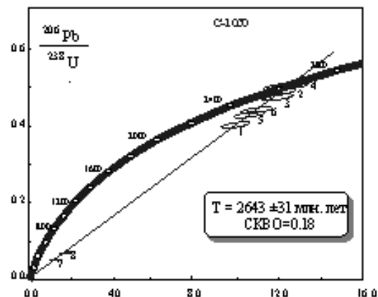
Рис. 3. Диаграмма с конкордией для цирконов из анортозитов массива Маристый
