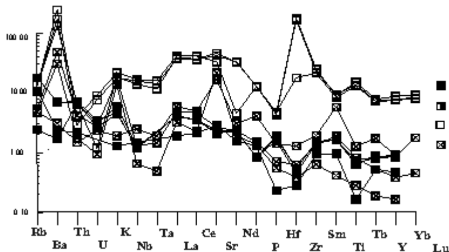
Рис. 4 Нормированные по первичной мантии (Sun, Donogh, 1989) спектры распределения малых элементов в породах Каларской группы массивов. Условные обозначения: 1 - 5 породы Каларской группы массивов: 1 - перидотиты, серпентиниты; 2 - пироксениты; 3 - габброиды; 4 - анортозиты;
