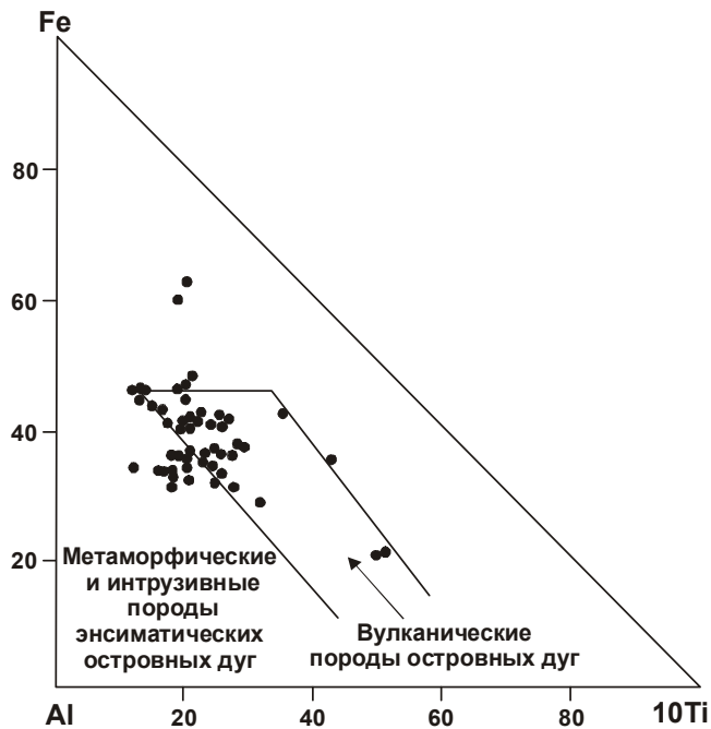
Рис. 8. Диаграмма состава обломочных амфиболов из песчаников р. Кемы и их вероятных вулканических источников [35].
