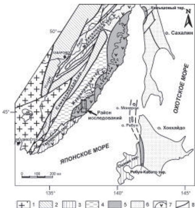
Рис. 1. Схема терреинов юга Дальнего Востока России и прилегающих территорий [6, 20].
