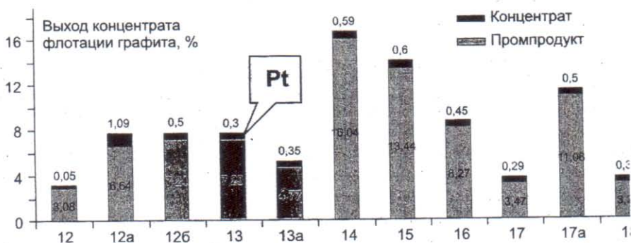
Рис. 4. Флотация графита. Общая исходная проба. 12 – без реагента; 12а – контрольная флотация с сосновым маслом; 126 – основная и контрольная флотации без реагентов; 13 – с керосином (3 перечистки); 13а – контрольная флотация с сосновым маслом; 14 – с сосновым маслом и керосином; 15 – с сосновым маслом и керосином, CaO, pH 10; 16 – с сосновым маслом и керосином, H 2 SO 4 , pH 4,7; 17 – 1-я стадия без реагента; 17а – 2-я стадия с керосином и сосновым маслом; 18 – с сосновым маслом, керосином, клеем
