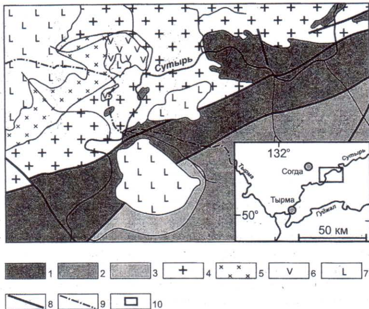
Рис. 1. Геологическая схема района работ. 1 – Сутырская толща (PR); 2 – Эпиканская свита ( J_2 ); 3 – Ургальская серия ( J_3-K_1 ); 4 – граниты Суларинского комплекса; 5, 6 – Тырмо-Бурейнский комплекс: 5 – граниты, гранодиориты, 6 – габбро, диориты; 7 – базальты Аякитской толщи ( N_1 ); 8 – разломы; 9 – лесовозная дорога; 10 – район работ (на врезке)
