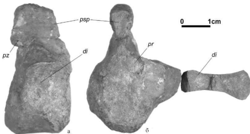
Рис. 4. Хвостовой позвонок Plesiosauria indet. (экземпляр ЗИН РН 1/48) сбоку (а) и спереди (б). Ново-нежино; Приморский край, кангаузская свита, верхний альб. Правый поперечный отросток отсутствует, левый поперечный отросток частично разрушен, его положение восстановлено по отпечатку на породе; di – поперечный отросток; pr – презигапофиз; psp – остистый отросток; pz – постзигапофиз
