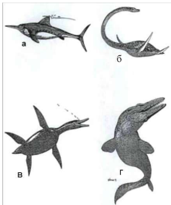
Рис. 1. Реконструкция: а – ихтиозавр, б – с длинной шеей плезиозавр ( elamosaurid ), в – с короткой шеей плезиозавр ( Pliosaurid ), г – мазозавр ( Mosasaur ). Животные б, г являются крупнейшими (достигают до 12 м), а, в – от 3 до 4 м [20]
